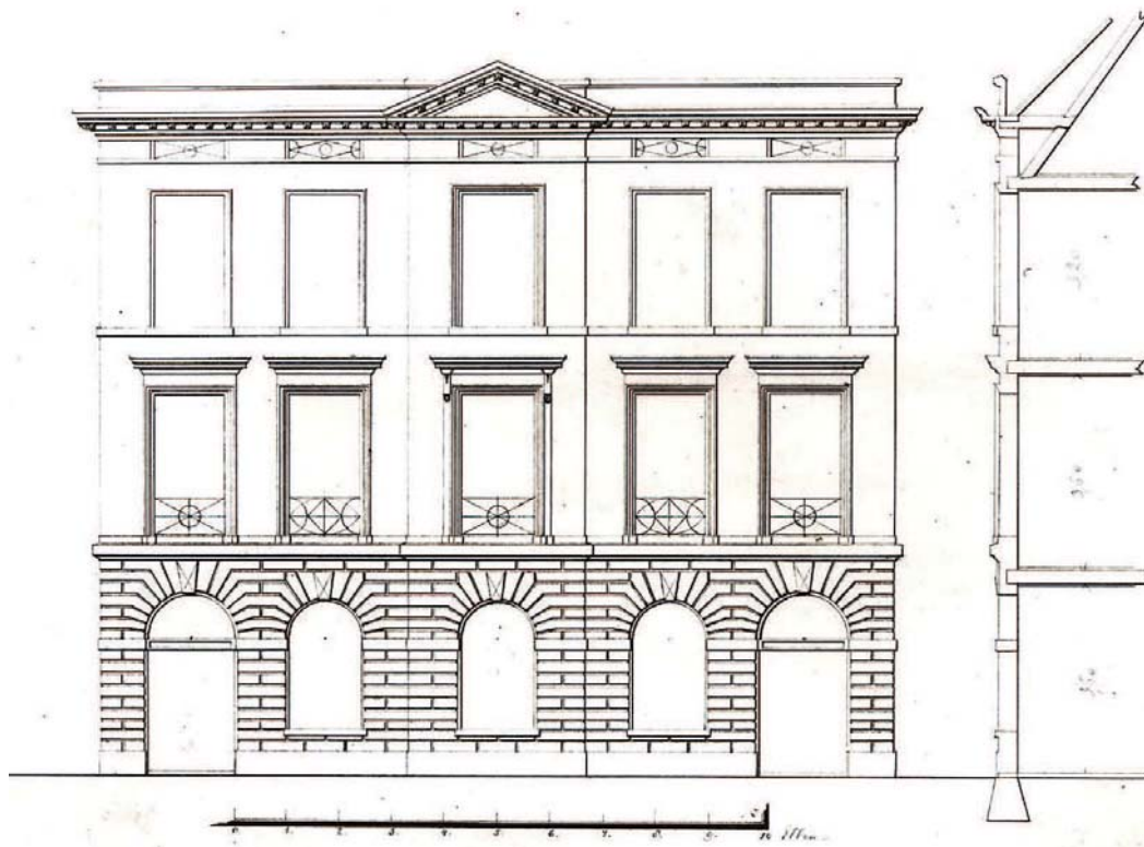
Afb. 14 Definitieve ontwerp voor nieuwe gevel van het Weeshuis aan de Oudegracht uit 1838 door F.C.E. van Embden. (Herkomst: HUA, Weeshuisarchief, inv. 24, nr. 238).
