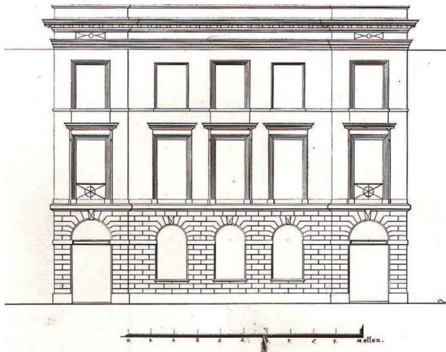
Afb. 13 Derde ontwerp voor nieuwe gevel van het Weeshuis aan de Oudegracht uit 1838 door F.C.E. van Embden. (Herkomst: HUA, Weeshuisarchief, inv. 24, nr. 238)
