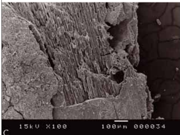
Afb. 6.18: SEM-foto van verkoold residu aangekoekt op scherf LR06 (vnr. 292/250) (foto's: L. Kubiak-Martens, BIA Consult).
