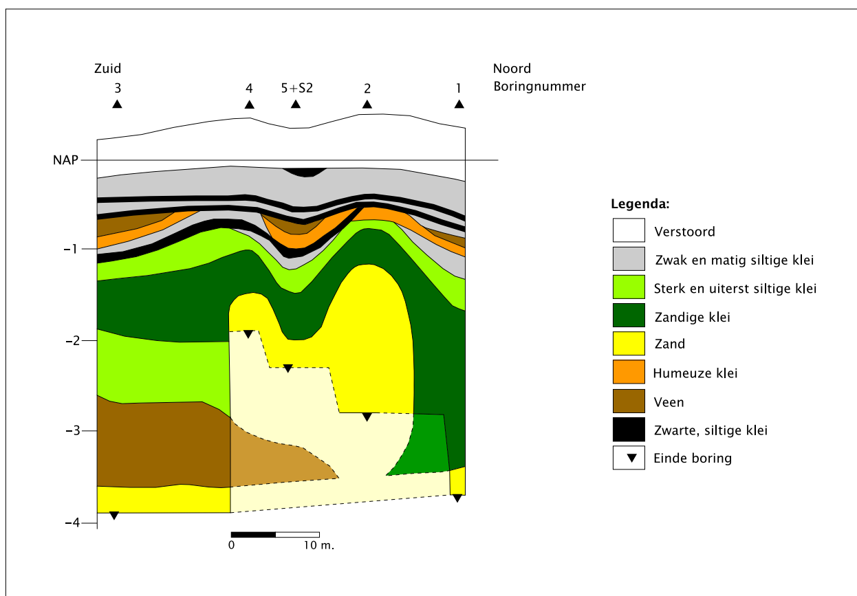
Afb. 2.4: Opbouw van de ondergrond ter hoogte van werkput 27.
