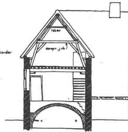
DOORSNEDE AB
