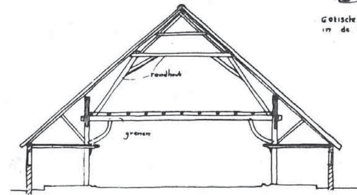
DOORSNEDE EF
