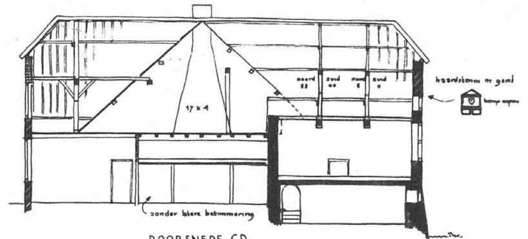
DOORSNEDE CD
