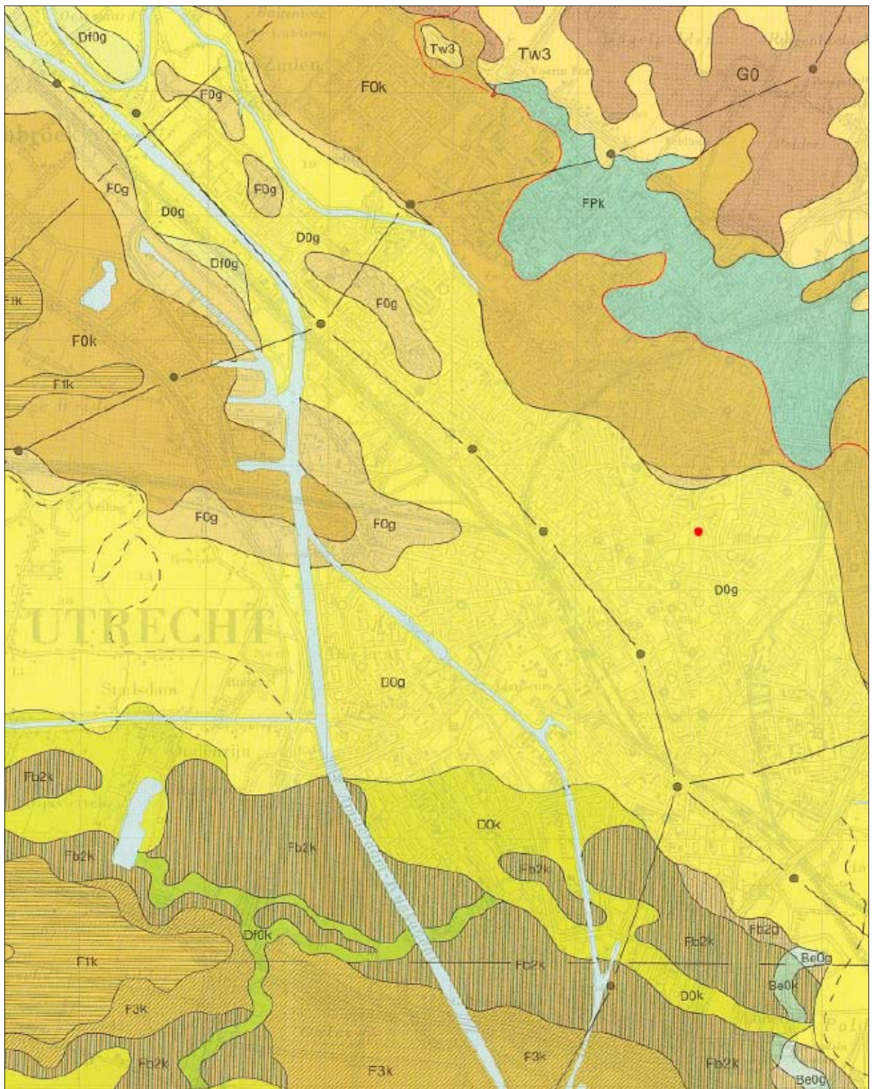
Afb. 2.1 De ligging van het plangebied op de bodem- en geomorfologische kaart (bron: Van de Meene et al , 1988).
