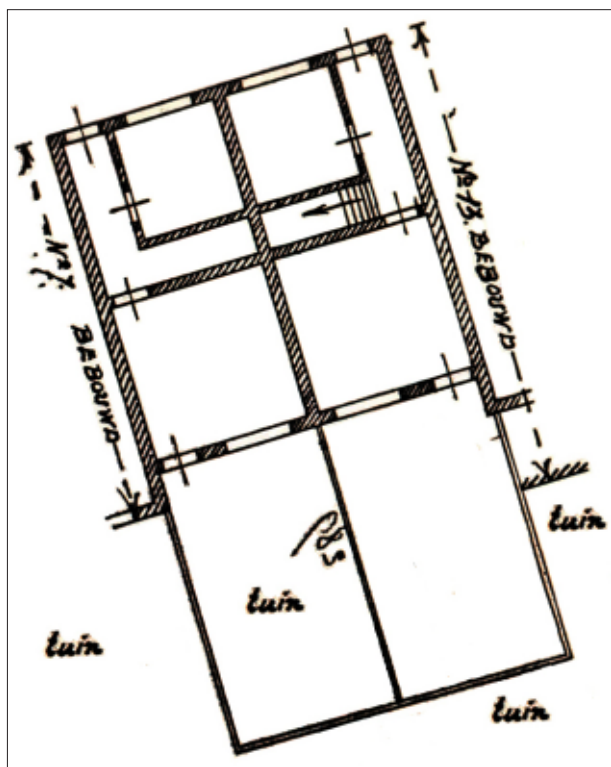
Afb. 4.5 Opmeting van Molenstraat 9 en 11 voorafgaand aan de bouw van het pakhuis met bovenwoningen in 1922.
