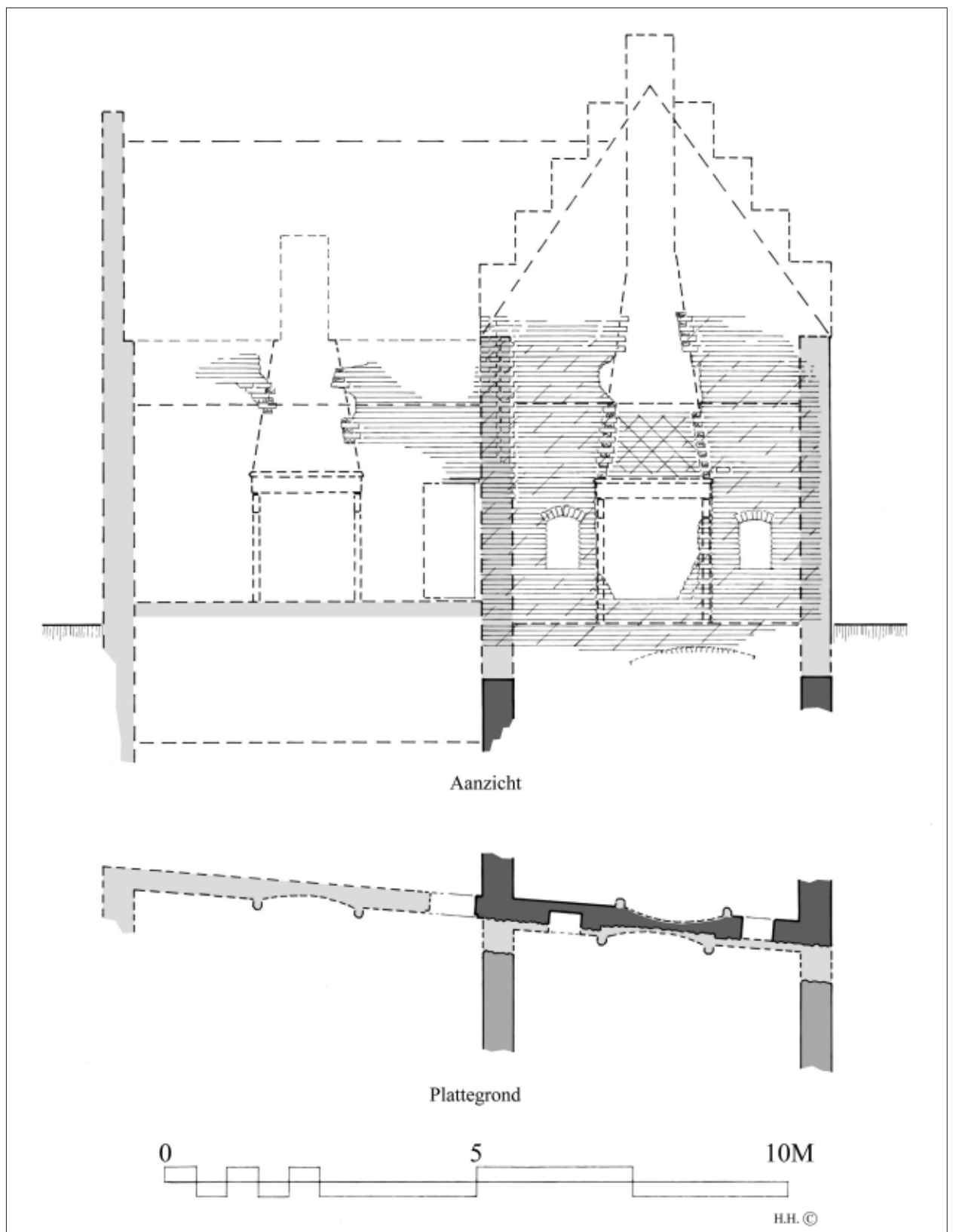
Afb. 4.6 Documentatietekening van het aanzicht en plattegrond van de van oorsprong gemeenschappelijke gevel tussen Molenstraat 3 en Plompentorengracht 13 en de zijgevel van de achtervleugel van Molenstraat 3. In het aanzicht is het middeleeuwse metselwerk aangegeven, met een arcering het afgehakte metselwerk en met een kruisarcering de beroete achterwand van de oorspronkelijke schouwboezem. Met stippellijnen zijn de oorspronkelijke schouwen, vloerniveaus, nissen, doorgang, rookkanaal en trapgevel aangegeven. Met een donkere grijze kleur is de doorsnede van het bewaard gebleven muurwerk aangegeven en met een lichtgrijze kleur de reconstructie van het muurwerk en keldergewelf.
